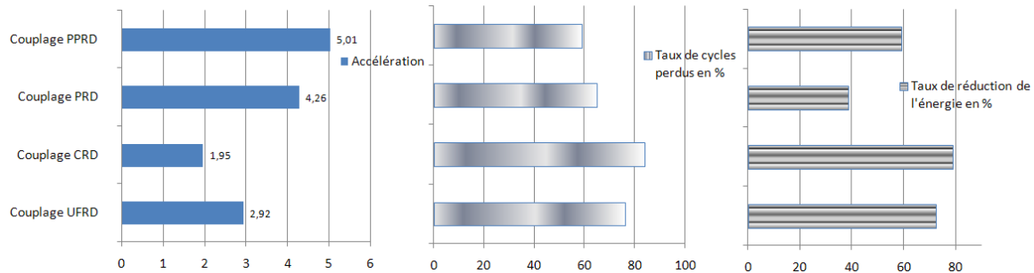
Figure 4-14 – Performances de l'architecture hybride DART/TMS320C6713 pour les différents couplages pour la tâche 3 de la phase "tracking". Le couplage PPRD présente la meilleure accélération de calcul : 5 fois contre 1.95 fois pour le couple PRD. Le couplage CRD présente un meilleur taux de réduction de la dissipation d'énergie (78.9%).
