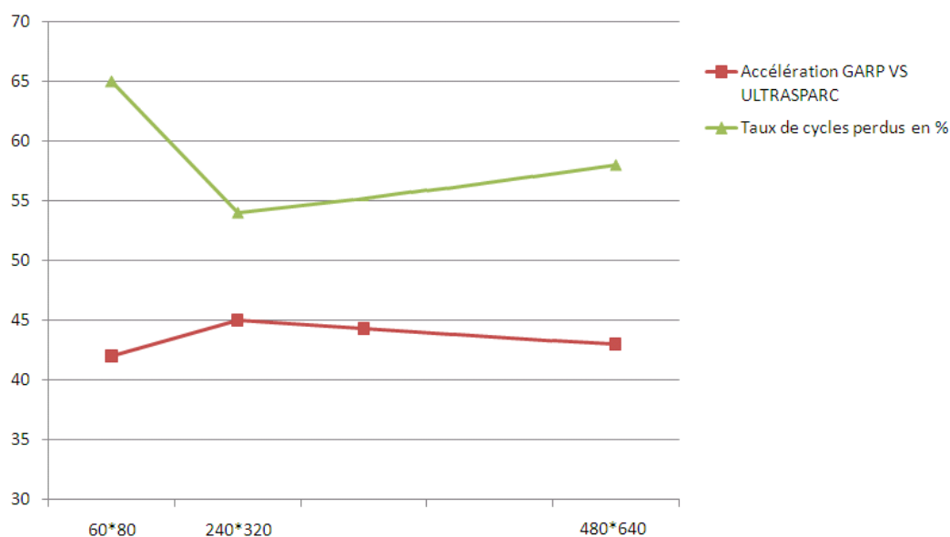
Figure 2-8 – Taux de cycles perdus et accélération de l'architecture hybride GARP (par rapport au processeur ULTRASPARC) en fonction de la taille d'image en pixels. Le taux de cycle perdus diminue d'autant que la taille d'image en pixels est plus grande et il sature à 58%. Une accélération entre 35 et 42 par rapport aux performances de l'ULTRASPARC est à souligner.
